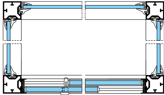
MOBILIER VITRINE AVEC PORTE COULISSANTE
