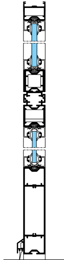
PORTE BATTANTE OUVERTURE EXTÉRIEURE
