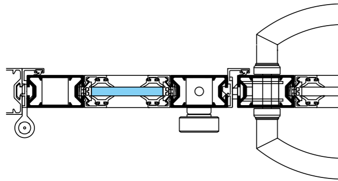
PORTE 2 VANTAUX SUR PAUMELLES
