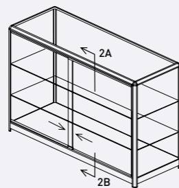
Module 24 mm
