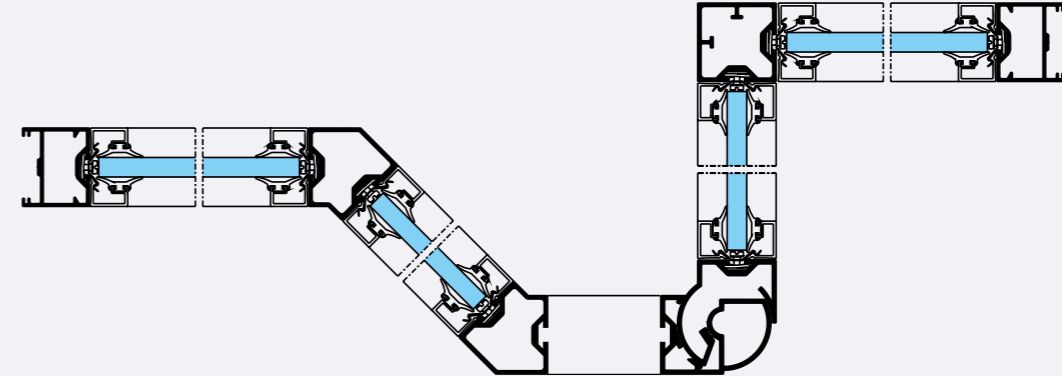
SYSTÈME TECHNAL DEVANTURE À ANGLE VARIABLE
